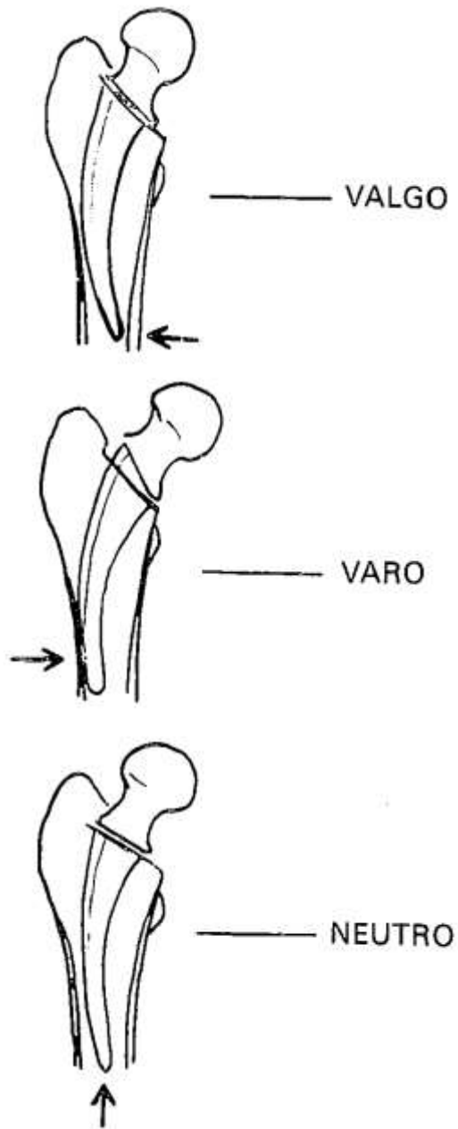
Figura 3. Representación esquemática de la situación del vástago en el interior de la cavidad diafisaria femoral (valgo, varo y neutro).
