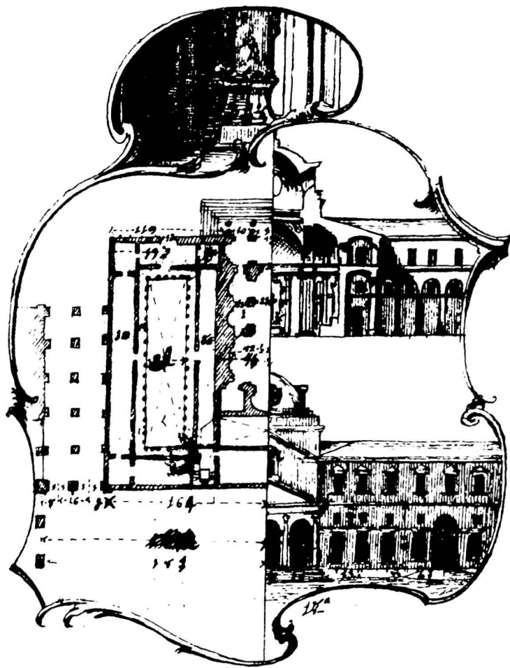
Fig. 8. Diego de Villanueva. Croquis de la planta, alzado y secciones de la iglesia del puerto.
