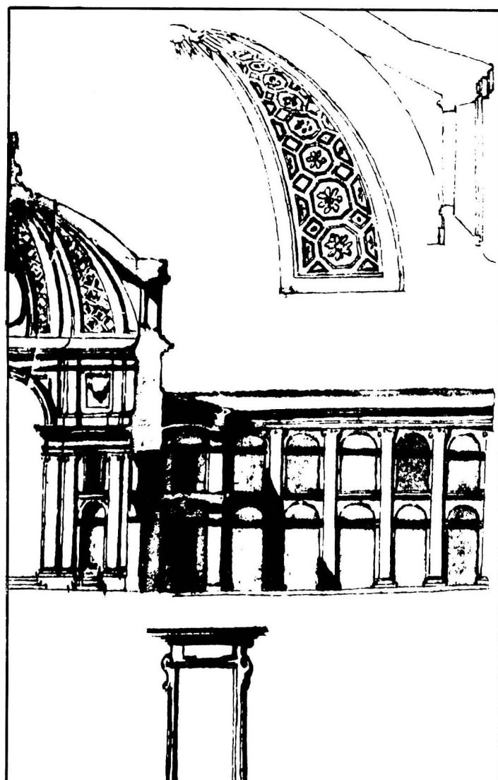
Fig. 2. Diego de Villanueva. Sección lateral de la iglesia.
