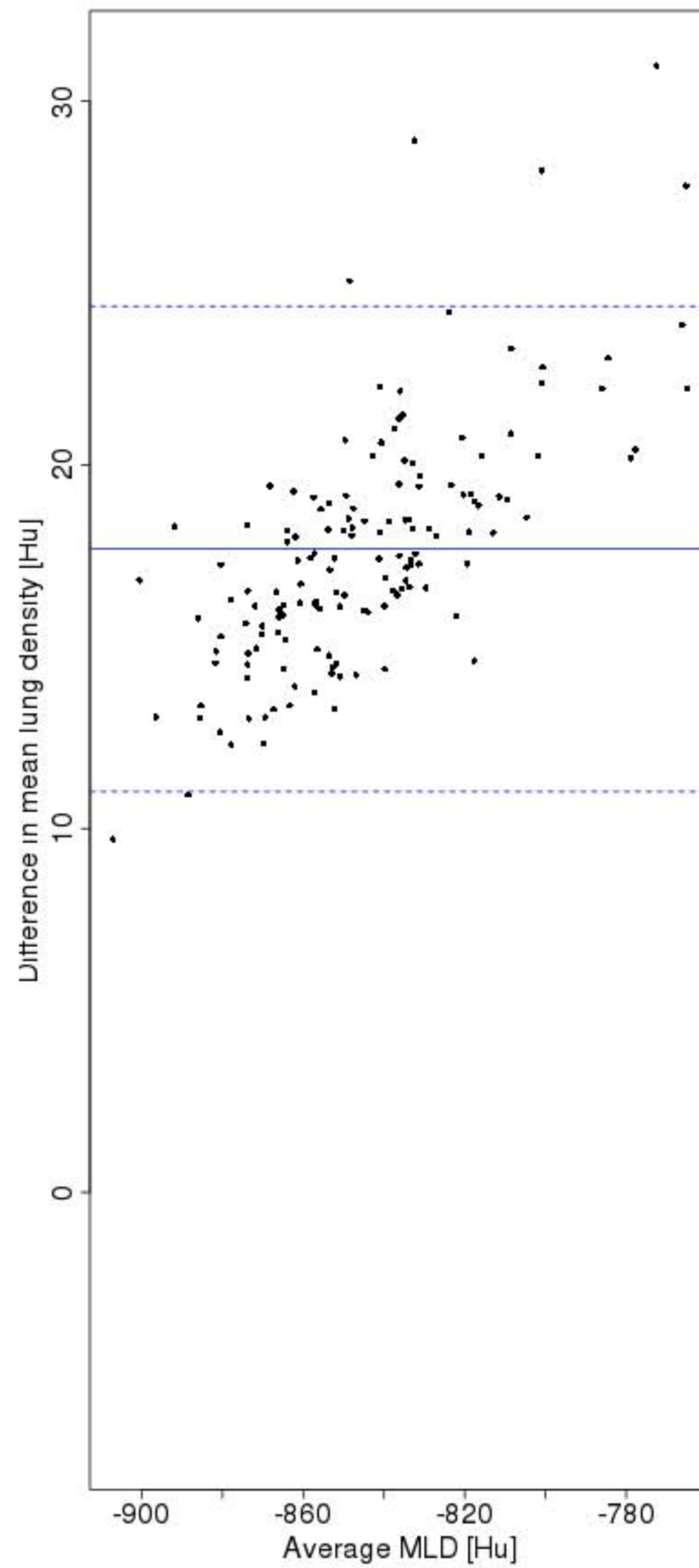
MLD
